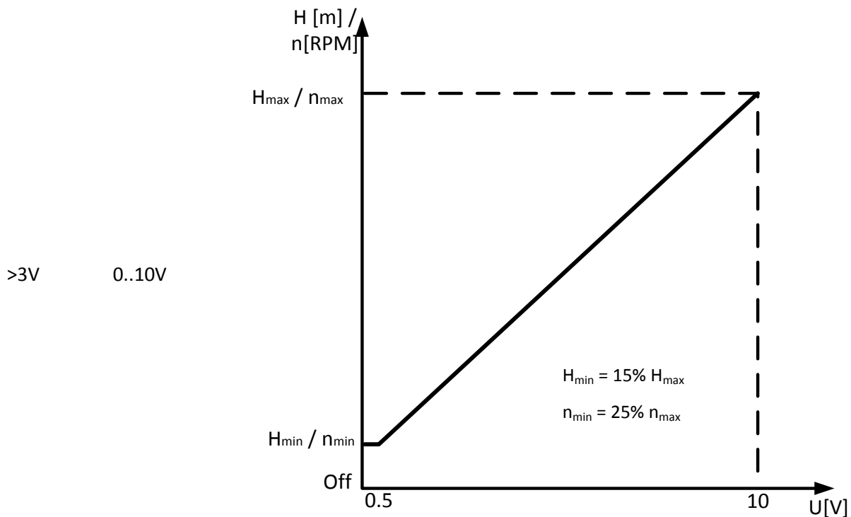
4. ábra: Külső 0..10V szabályozási jelleggörbe
