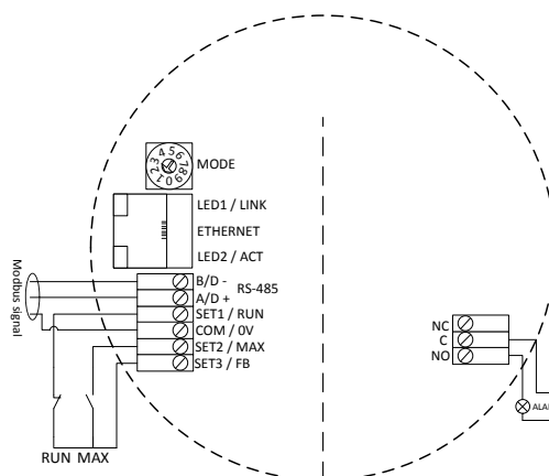
1. ábra: Tipikus modul csatlakozás
